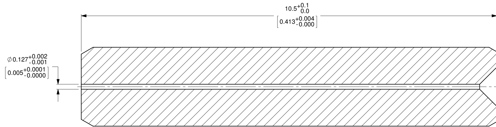
SECTION A-A
