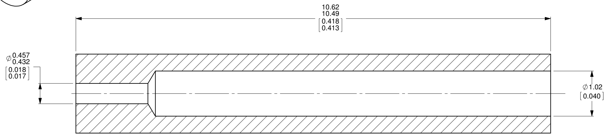
SECTION A-A
