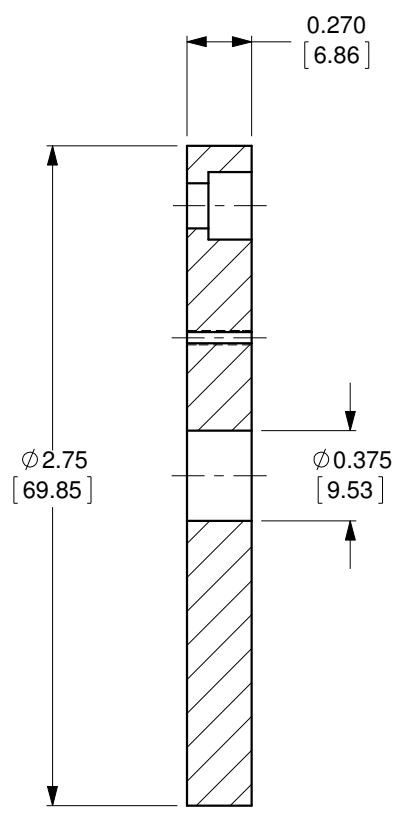
SECTION A-A
