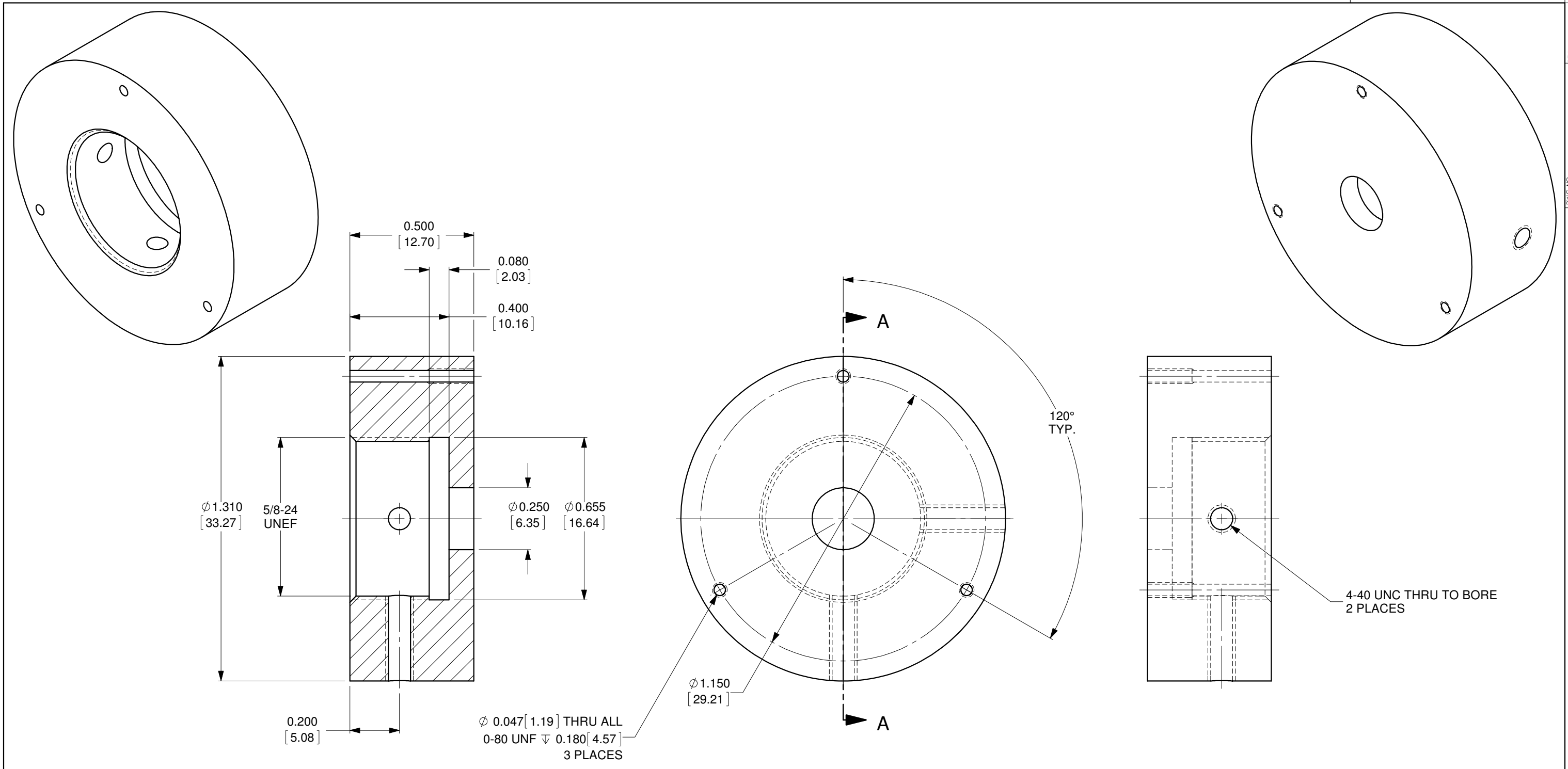
SECTION A-A
